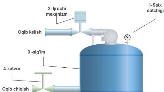
1.1-rasm. Suyuqlik oqib kelishi va oqib chiqishiga ega bo'lgan sig'im sathini avtomatik tarzda rostlash: 1 – satx datchigi ; 2 – ijrochi mexanizm; 3 – sig'im; 4 – zatvor.
