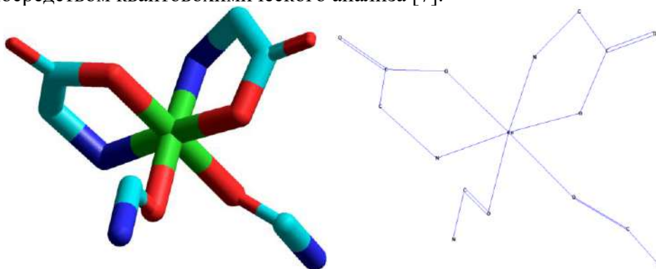
Рис.1. Пространственное строение молекулы [Cu(Gl-H) 2 2FA]
