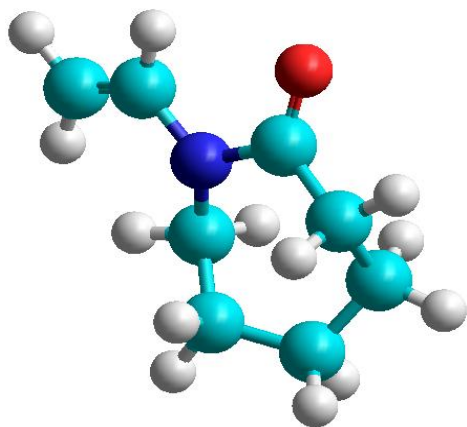
1-rasm. N-vinilkaprolaktam molekulasi-ning fazoviy tuzilishi
