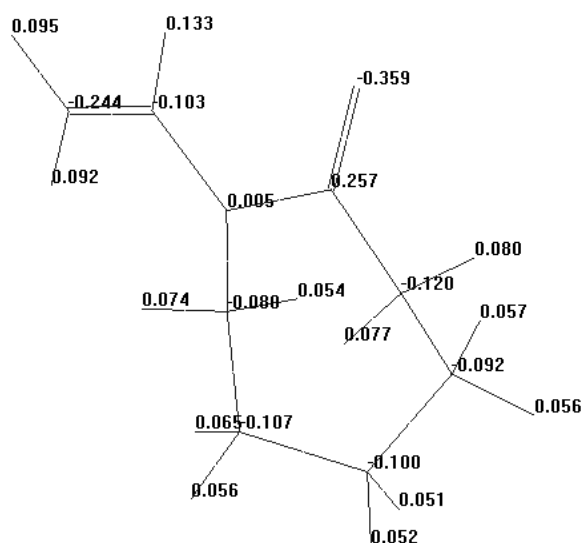
2-rasm. N-vinilkaprolaktam molekulasida elektron zaryadlar qiymati
