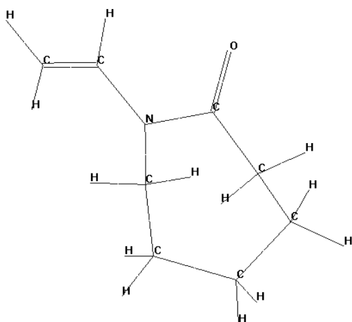
4-rasm. N-vinilkaprolaktamning atomlararo bog` uzunliklari fazoviy tuzilishi
